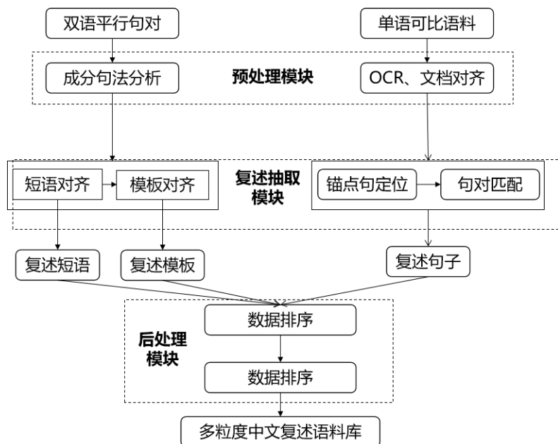
图1 复述抽取系统总体框架
