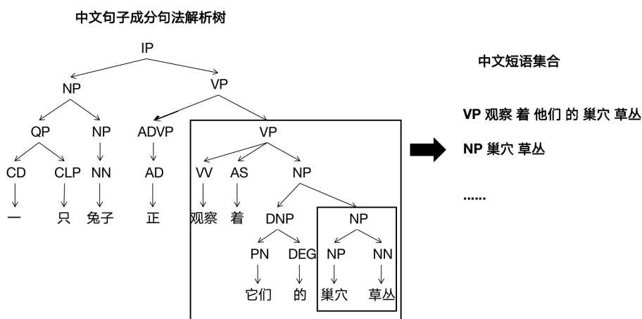
图2 短语抽取实例
