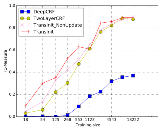
图9 特征变换方法 TransInit 实验结果 [25]
