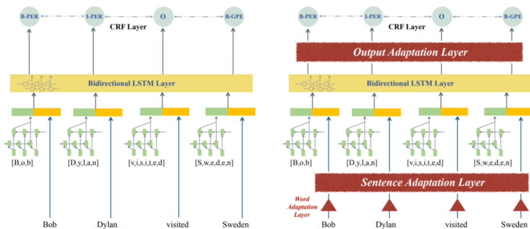
图 10 跨域模型对比 [26]
